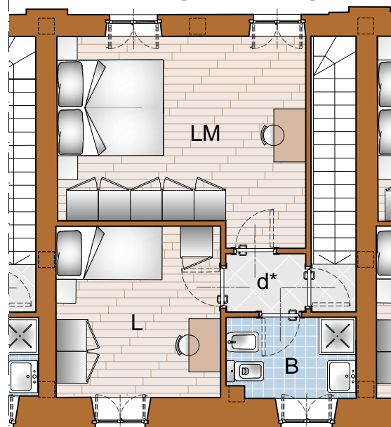
PIANO PRIMO
